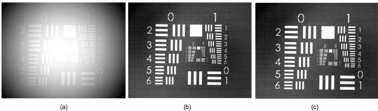
그림 8. USAF를 이용한 적외선 영상 표적 식별, (a) 적외선 원 영상, (b) 불균일보정을 수행한 적외선 영상, (c) 불균일보정과 불량픽셀보정을 수행한 적외선 영상
