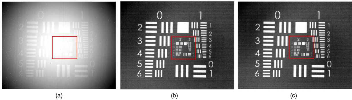
그림 9. USAF를 이용한 적외선 영상의 분해능, (a) 적외선 원 영상, (b) 불균일보정을 수행한 적외선 영상, (c) 불균일보정과 불량픽셀보정을 수행한 적외선 영상 Fig. 9. Resolution of infrared images using USAF, (a) Infrared original image, (b) Infrared image performed with non-uniformity correction, (c) Infrared image performed with non-uniformity correction and defective pixel correction
