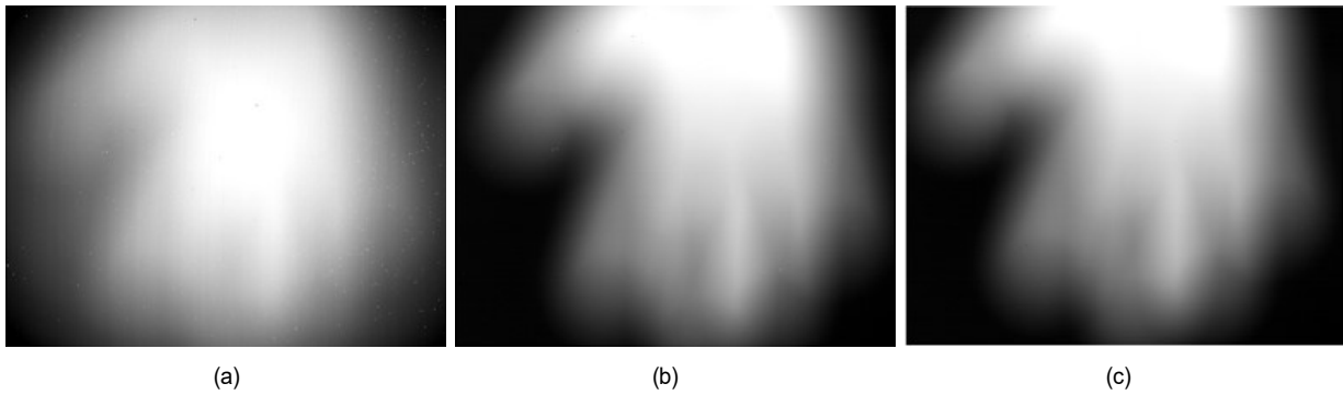
그림 7. 실험 참가자의 손을 식별한 적외선 영상, (a) 적외선 원 영상, (b) 불균일보정을 수행한 적외선 영상, (c) 불균일보정과 불량픽셀보정을 수행한 적외선 영상
